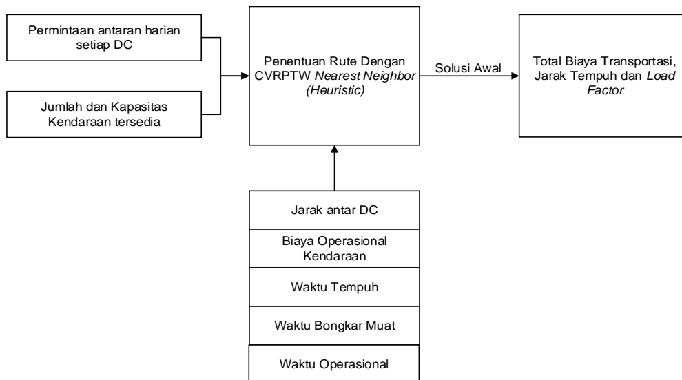
Gambar 2. Kerangka Konseptual
